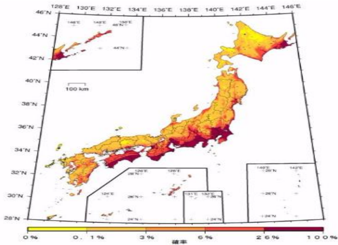
確率的地震動予測地図：確率の分布 今後30年間に震度6弱以上の揺れに見舞われる確率 (平均ケース・全地震)
